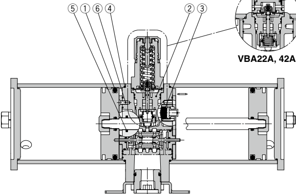
VBA20A, 22A, VBA40A, 42A, 43A
